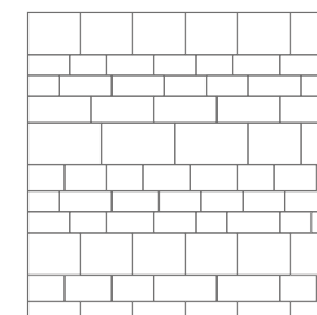
PATROON 5 Banenverband 20, 25 en 40 cm ca. 27% 20 cm ca. 33% 25 cm ca. 40% 40 cm
